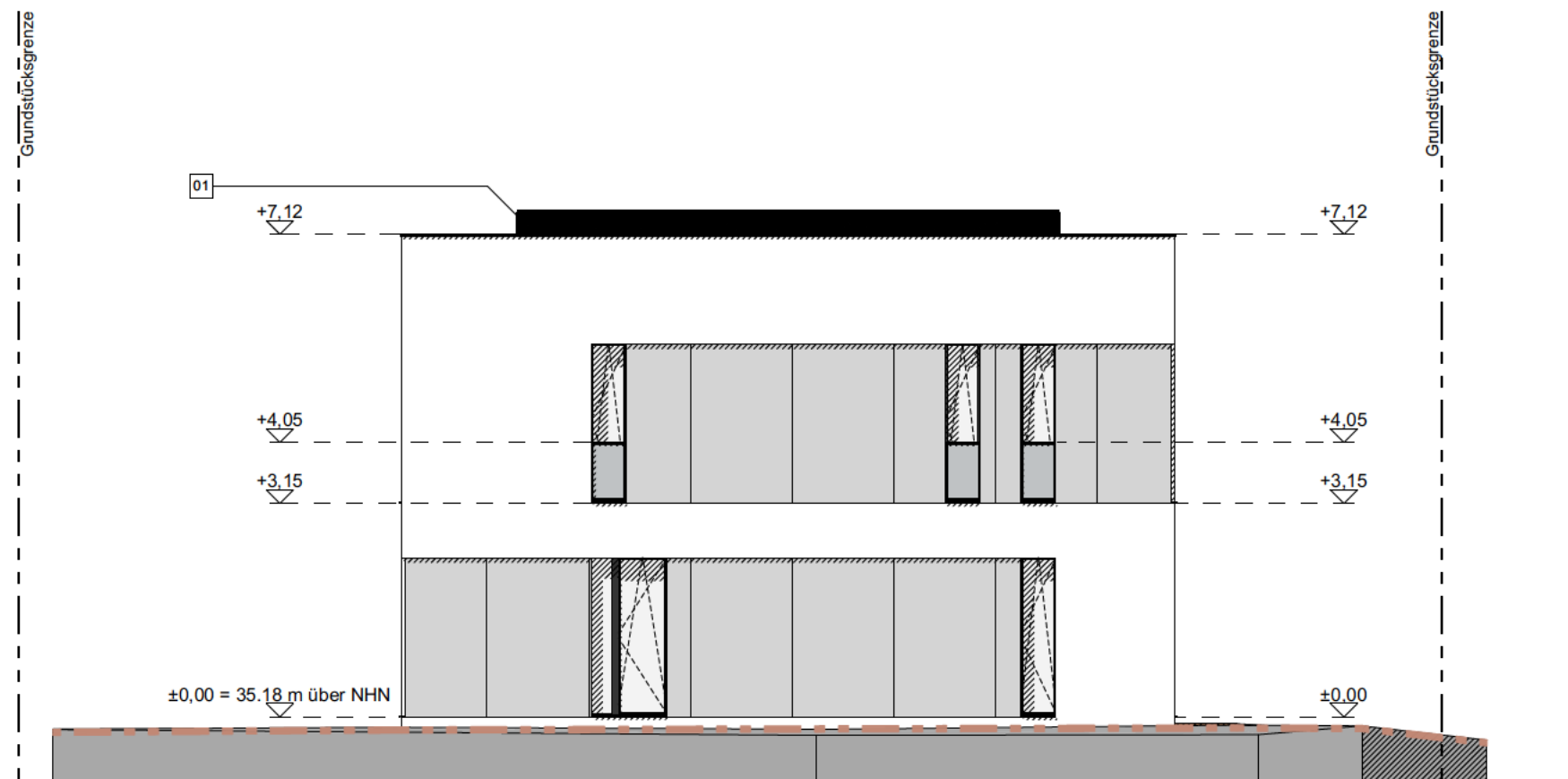
Ansicht Nord
