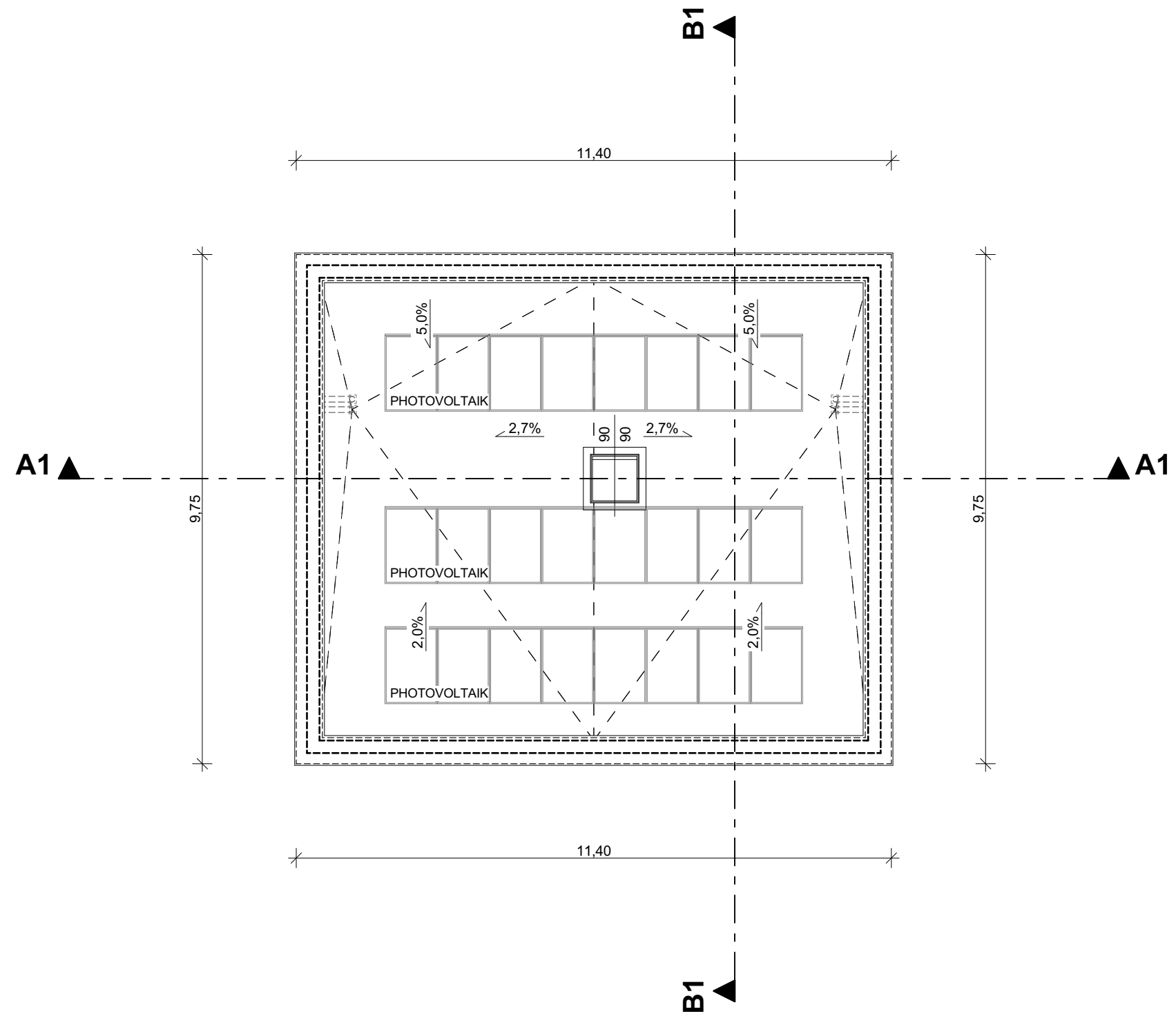
Dachaufsicht
