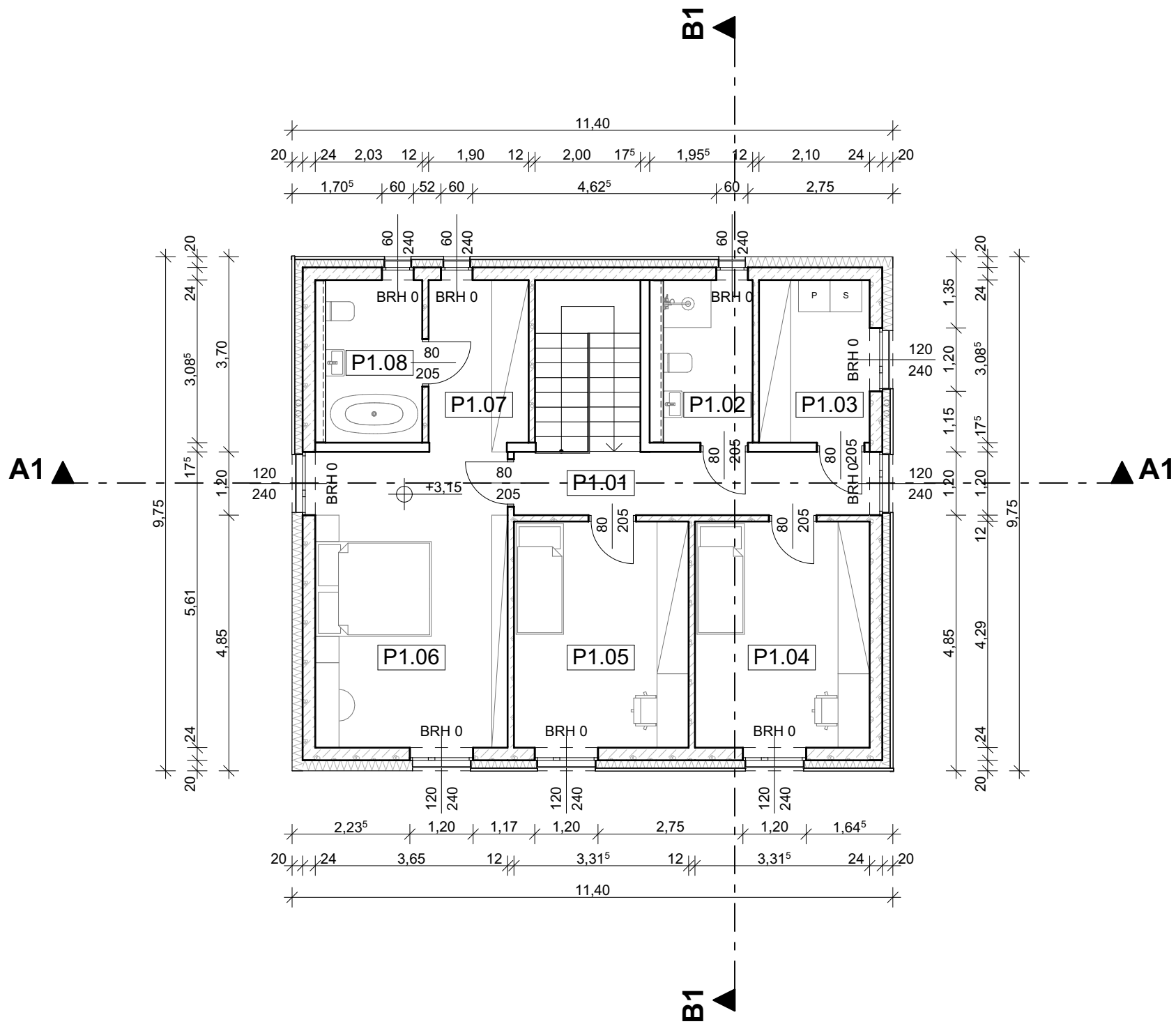
Obergeschoss
